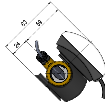
Komplet MULTICAL® 302 med regneværk monteret på flowdel
