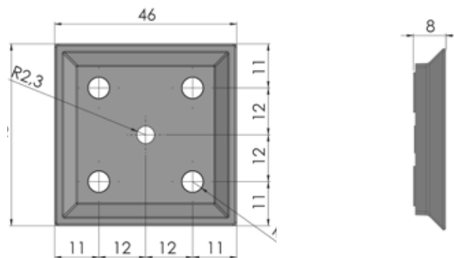
Vægbeslag til regneværk
