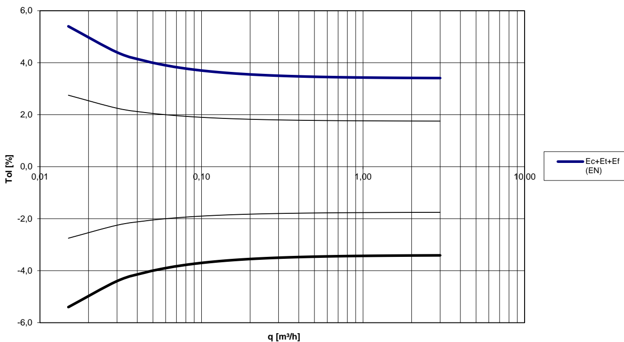
Diagramm 1: Typische Genauigkeit des MULTICAL® 402 im Vergleich zu EN 1434-1.
