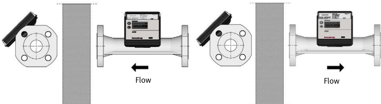
Abbildung 13: Flanschzähler
