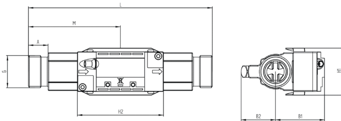
Abbildung 3: Durchflusssensor mit G 3/4 und G1 Gewindeanschluss
