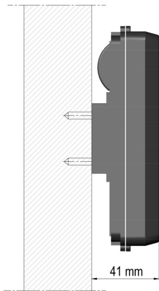
Abbildung 14: Wandmontage von MULTICAL® 402
