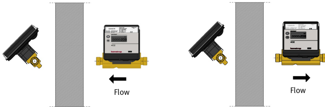
Abbildung 11: Verschraubungszähler
