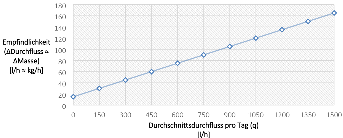
Leckagegrenze für \text{qp } 1,5 \text{ m}^3/\text{h} M-Code = 2 (1,0 % von qp + 10 % q)
