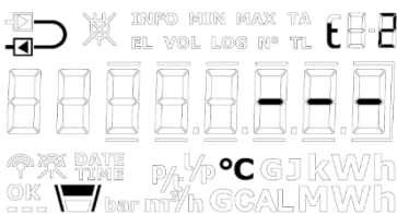
Anzeige von t2 bei Temperaturfühlerfehlern.
