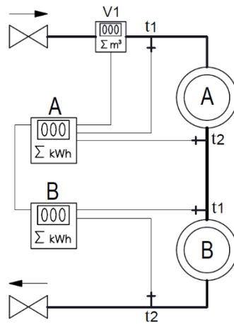
Abb. 11 Wärmearanlage mit einem Durchflusssensor und 2 Rechenwerken.
