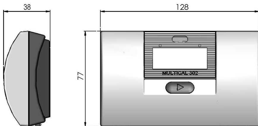
Vægmonteret regneværk
