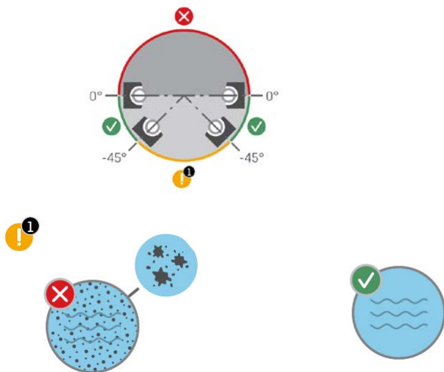
Figur 3. Acceptabel orientering af Kamstrups flowsensorer omkring røraksen i varmeinstallationer ved vandret montering. Målerhuse med gevind med q_p \leq 2,5 \text{ m}^3/\text{h} .
