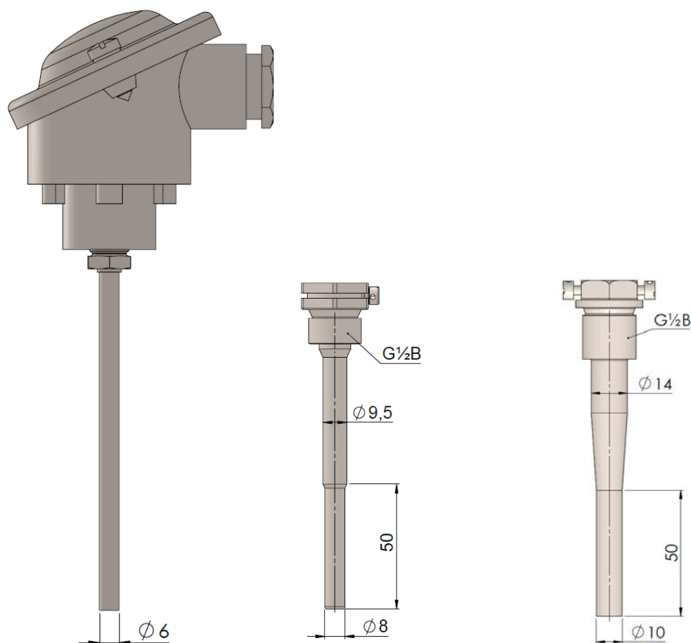
Figur 12: \varnothing 6 mm lommeføler med tilslutningshoved og tilhørende lommer.
