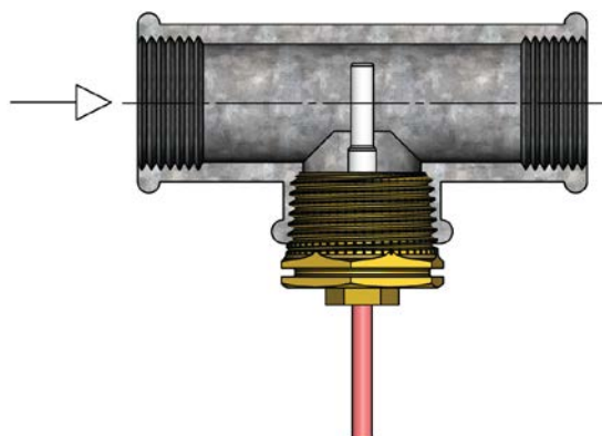
Figur 27: Kort direkte DS 27,5 mm temperaturføler monteret med nippel i et T-stykke.
