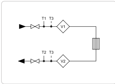
Exemple 1: Circuit de chauffage fermé avec 1 ou 2 mesureurs
