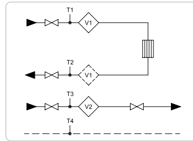
Exemple 2: Circuit de chauffage fermé avec deux mesureurs
