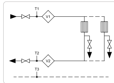
Exemple 4: Circuit ouvert avec deux mesureurs
