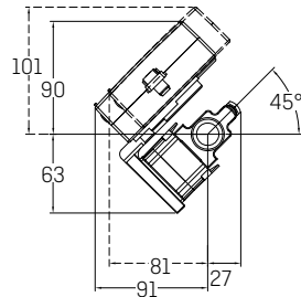
Montado en caudalímetro con accesorio de ángulo 3026-252
