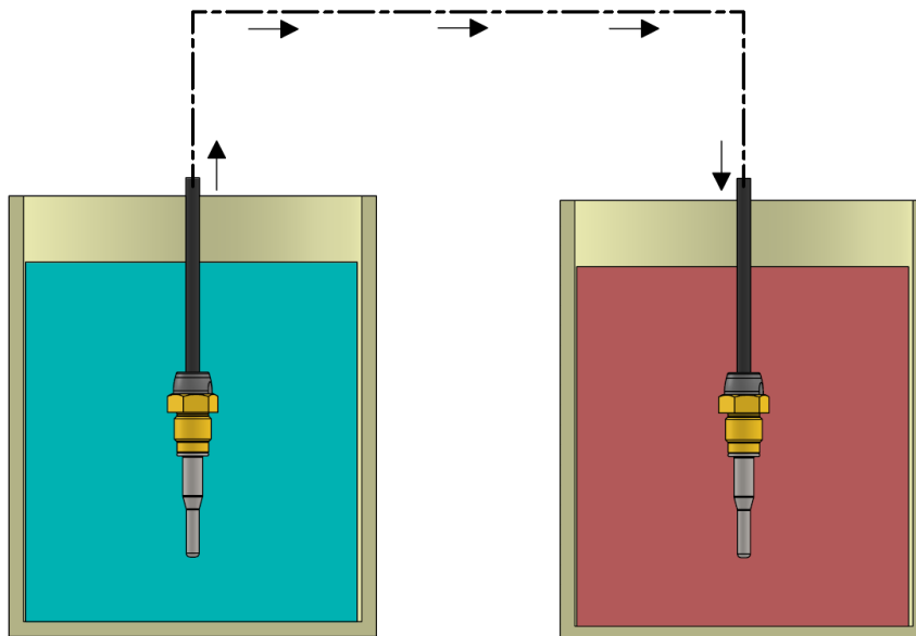
Abb. 16: Darstellung einer Einrichtung zur Messung der Reaktionszeit eines Temperaturfühlers, bei dem der Temperaturfühler von einem temperaturgeregelten Wasserbad in ein anderes temperaturgeregeltes Wasserbad umgesetzt wird. Der Temperaturunterschied zwischen den beiden Bädern beträgt normalerweise 10 K.
