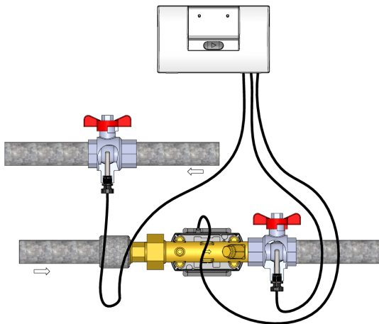
Abb. 22: Beispiele für eine symmetrische Installation und eine asymmetrische Installation.
