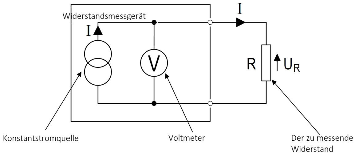
Abb. 3: Messung eines Widerstandswerts mit einer Konstantstromquelle und einem Voltmeter.
