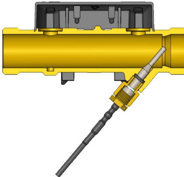
Abb. 35: Kurzer direkt eintauchender DS 38 mm Temperaturfühler montiert mit 11 mm Adapter in einem Durchflusssensor.
