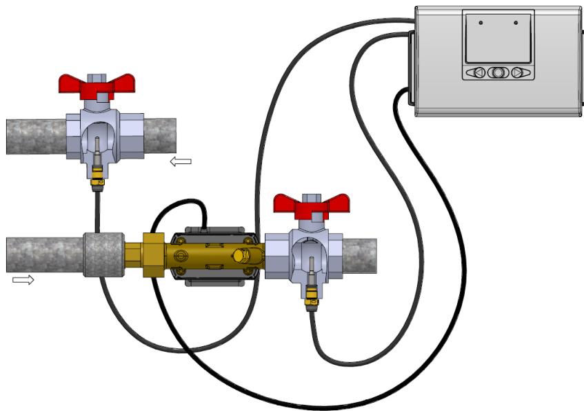
Abb. 21: Typische Installation eines Wärme- oder Kältezählers, in welcher ein Temperaturfühler im Vorlauf und ein Temperaturfühler im Rücklauf installiert sind.
