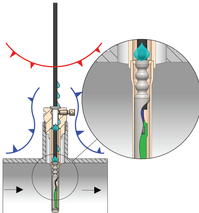
Abb. 36: Eindringen von Kondenswasser in einen Tauchhülsefühler.
