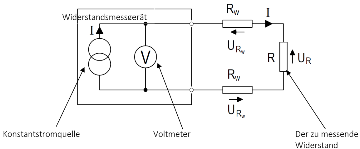
Abb. 4: Einfluss der Kabel auf den gemessenen Widerstandswert.
