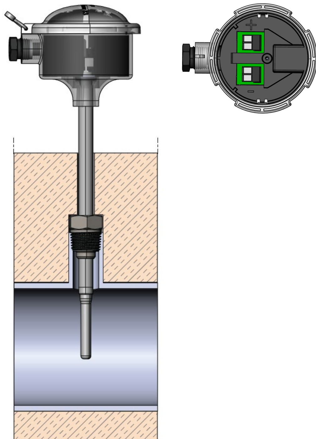
Abb. 13: \varnothing 5,8 mm Tauchhülsenfühler mit Anschlusskopf, der in einem isolierten Rohr montiert ist.
