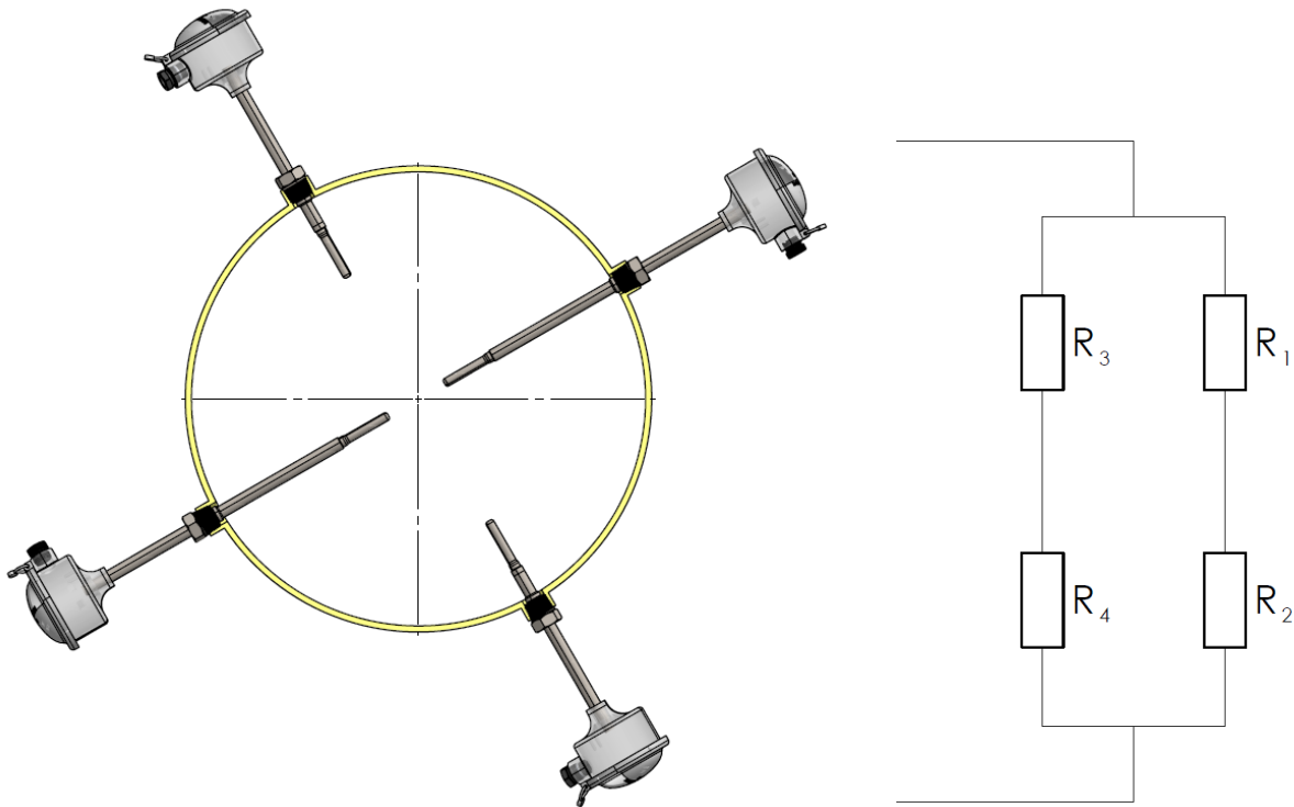
Abb. 26: Beispiel für eine Installation, bei der eine repräsentativere Durchschnittstemperatur durch die Verwendung von vier verschiedenen Temperaturfühlern erzielt wird, die durch eine Kombination aus Reihen- und Parallelschaltung miteinander verbunden sind.
