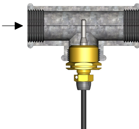
Abb. 24: Beispiel für die richtige Installation des kurzen direkt eintauchenden Temperaturfühlers.
