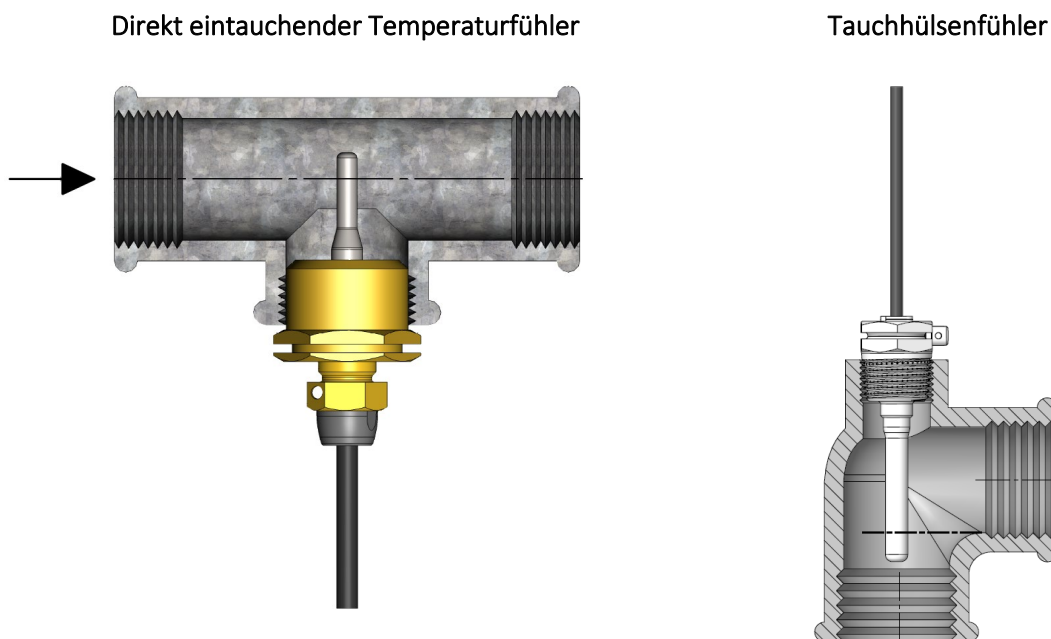
Abb. 8: Abbildung eines direkt eintauchenden Temperaturfühlers und eines Tauchhülsenfühlers.
