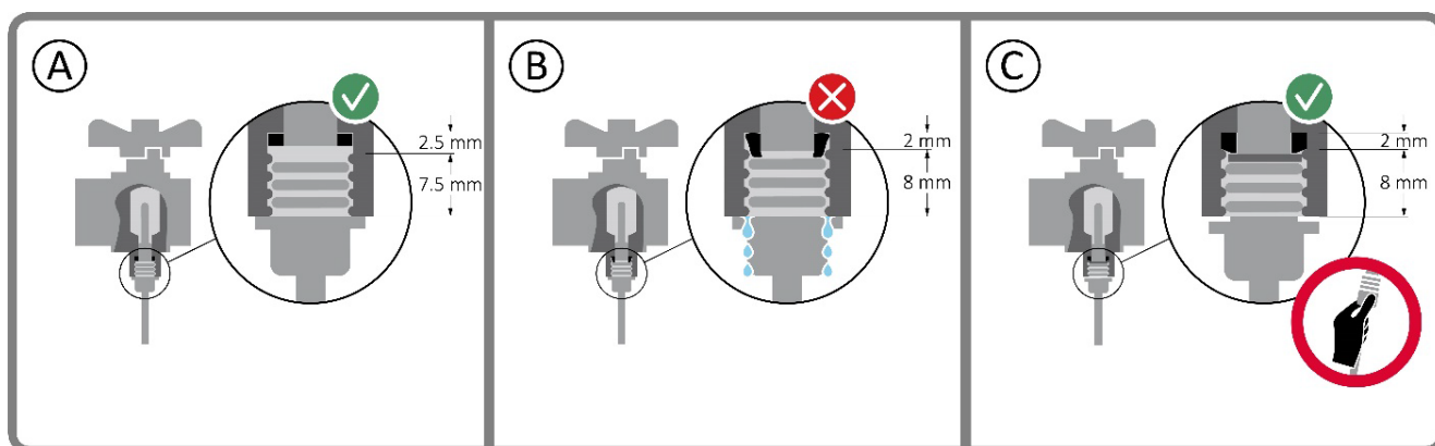
Abb. 32: TemperatureSensor 63 \varnothing 5,0 oder \varnothing 5,2 installiert in Kugelhahn (A) gemäß EN 1434:2022 oder (B), (C) gemäß früheren Versionen von EN 1434
