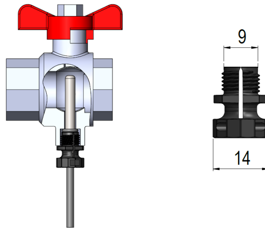
Abb. 12: \varnothing 5,2 mm Temperaturfühler mit Überwurfmutter aus einem Verbundwerkstoff, der in einem Kugelhahn montiert ist.
