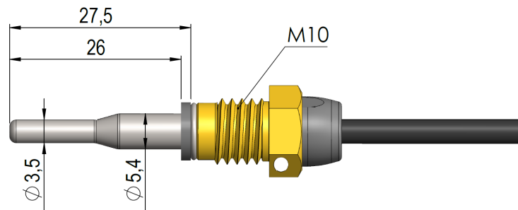
Abb. 9: Kurzer direkt eintauchender DS 27,5 mm Temperaturfühler.
