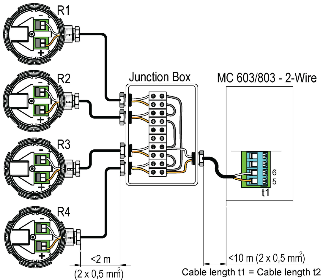
Abb. 27: Beispiel für eine Installation mit 4 Temperaturfühlern in einem Rohr. Die Installation wurde mit einem 2-Leiteranschluss durchgeführt, was die Kabellänge auf 10 m begrenzt. In diesem Beispiel wird der Anschluss von t1 (Vorlauffühler), der an das Rechenwerk MULTICAL® 603 angeschlossen ist, dargestellt. Eine entsprechende Installation muss für t2 (Rücklauffühler) durchgeführt werden.
