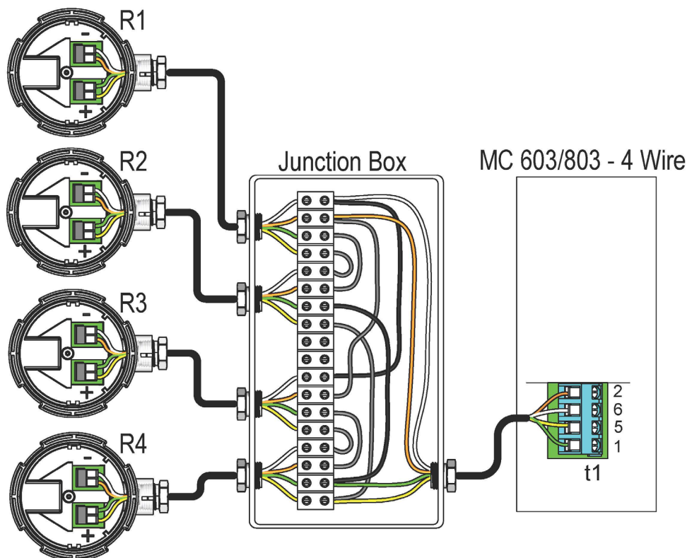
Abb. 29: Beispiel für eine Installation mit 4 Temperaturfühlern in einem Rohr. Die Installation besteht aus einer 4-Leiteranschlüssen, was eine Kabellänge von 100 m zwischen dem Rechenwerk und den Temperaturfühlern ermöglicht. In diesem Beispiel wird der Anschluss von t1 (Vorlauffühler), der an das Rechenwerk MULTICAL® 603 angeschlossen ist, dargestellt. Eine entsprechende Installation muss für t2 (Rücklauffühler) durchgeführt werden. Andere zugelassene Rechenwerke, z. B. MULTICAL® 803, können in gleicher Weise verwendet werden.
