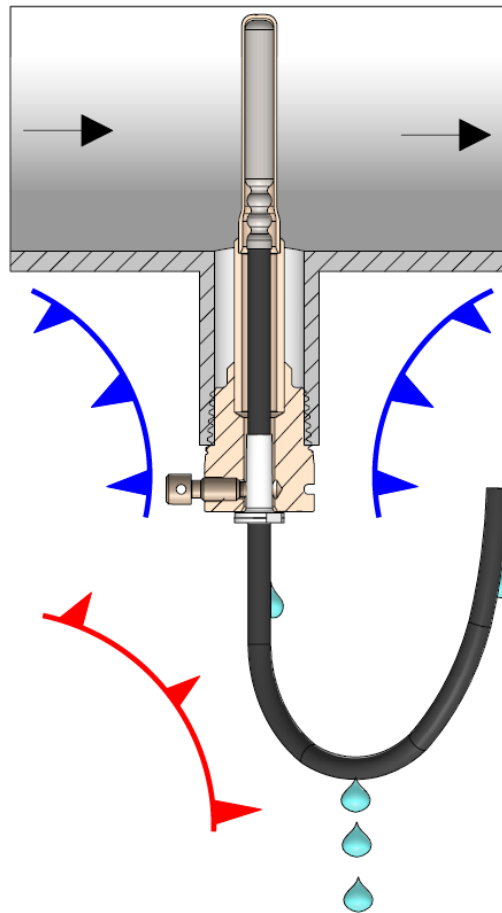
Abb. 38: Richtige Installation eines Temperaturfühlers für die Verwendung bei Kältemessungen, in denen durch die Schwerkraft das Eindringen von Kondensation verhindert wird.
