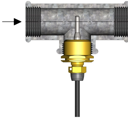
Abb. 33: Kurzer direkt eintauchender DS 27,5 mm Temperaturfühler montiert mit Rohrstück (Nippel) in einem T-Stück.
