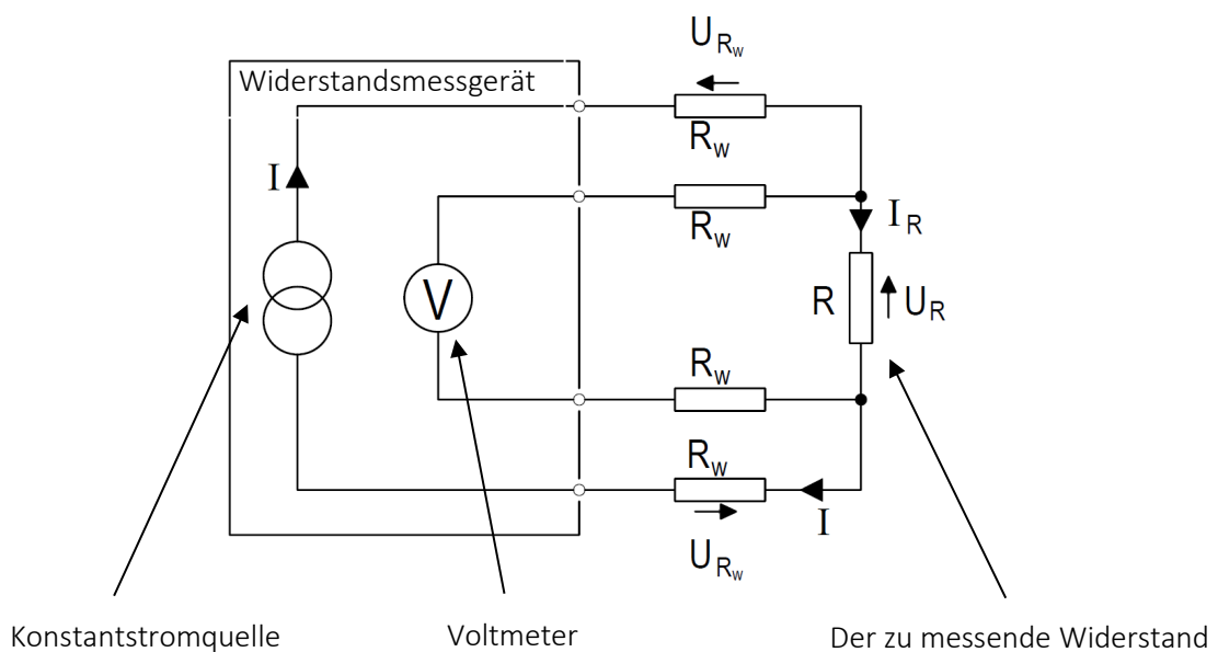
Abb. 5: Messung des Widerstandswertes nach dem 4-Leiterprinzip, bei dem die Kabel die Widerstandsmessung nicht beeinflussen.
