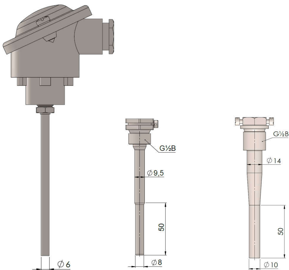
Abb. 14: \varnothing 6,0 mm Tauchhülsenfühler mit Anschlusskopf und entsprechenden Tauchhülsen.
