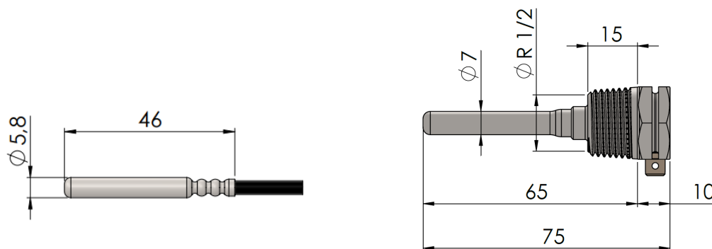
Abb. 10: \varnothing 5,8 mm Tauchhülsenfühler mit entsprechender 65 mm Tauchhülse.
