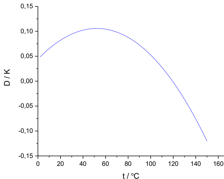
Abb. 20: Beispiel für eine Korrekturrechnung eines Pt500-Temperaturfühlers, bei der die Abweichung D von einem idealen Pt500-Temperaturfühler für alle Temperaturen t im Temperaturbereich 2-150 °C ermittelt wird.
