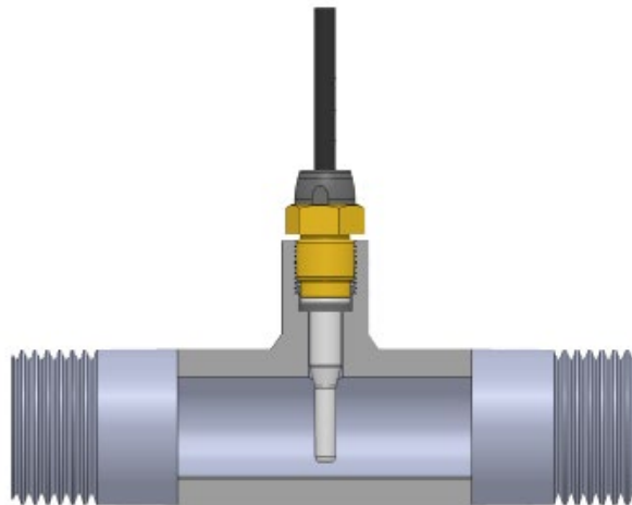
Abb. 34: Kurzer direkt eintauchender DS 27,5 mm Temperaturfühler montiert im T-Stück mit M10x1-Gewinde.
