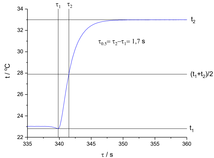
Abb. 15: Messung der Reaktionszeit eines kurzen direkt eintauchenden Temperaturfühlers.
