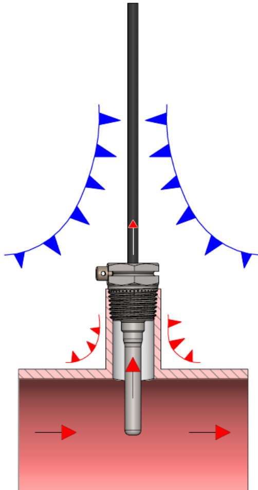
Abb. 17: Darstellung des Wärmeableitfehlers bei einer Temperaturmessung aufgrund der Wärmeableitung in die Umgebung.
