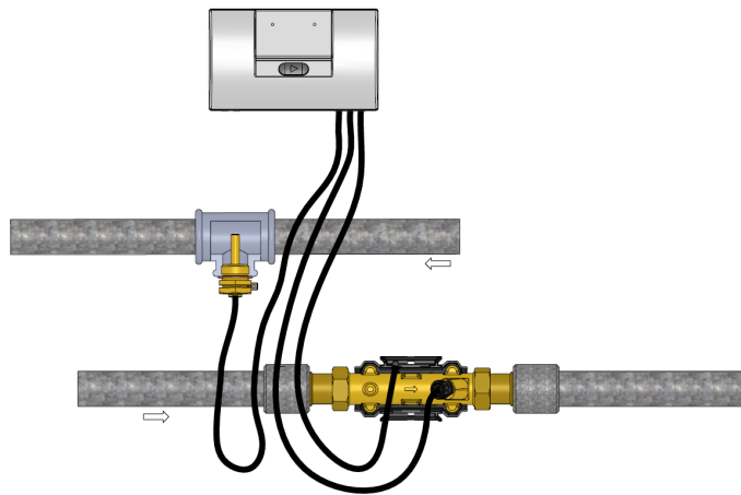
Abb. 22: Beispiele für eine symmetrische Installation und eine asymmetrische Installation.
