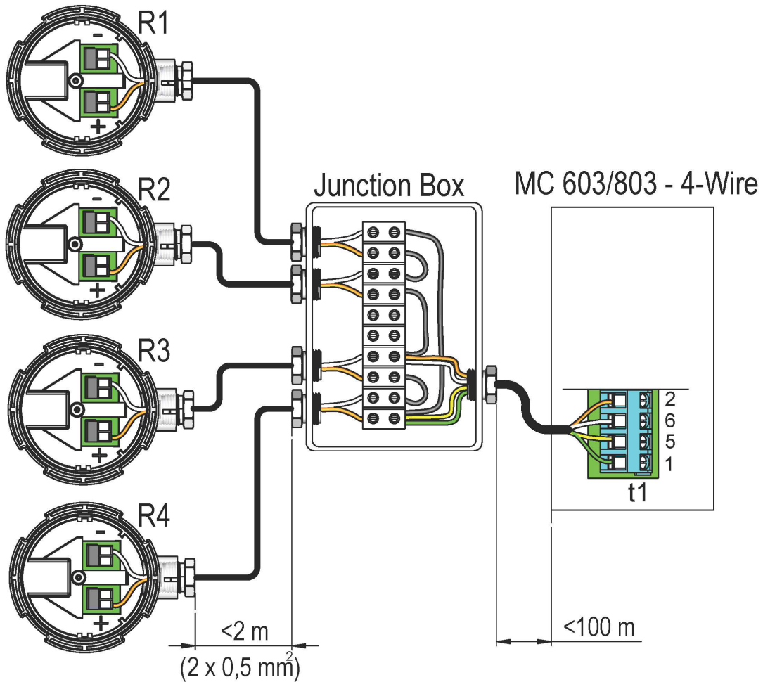
Abb. 28: Beispiel für eine Installation mit 4 Temperaturfühlern in einem Rohr. Die Installation besteht aus einer Kombination von 2-Leiter- und 4-Leiteranschlüssen, was eine Kabellänge von 100 m zwischen dem Rechenwerk und den Temperaturfühlern ermöglicht. In diesem Beispiel wird der Anschluss von t1 (Vorlauffühler), der an das Rechenwerk MULTICAL® 603 angeschlossen ist, dargestellt. Eine entsprechende Installation muss für t2 (Rücklauffühler) durchgeführt werden. Andere zugelassene Rechenwerke, z. B. MULTICAL® 803, können in gleicher Weise verwendet werden.
