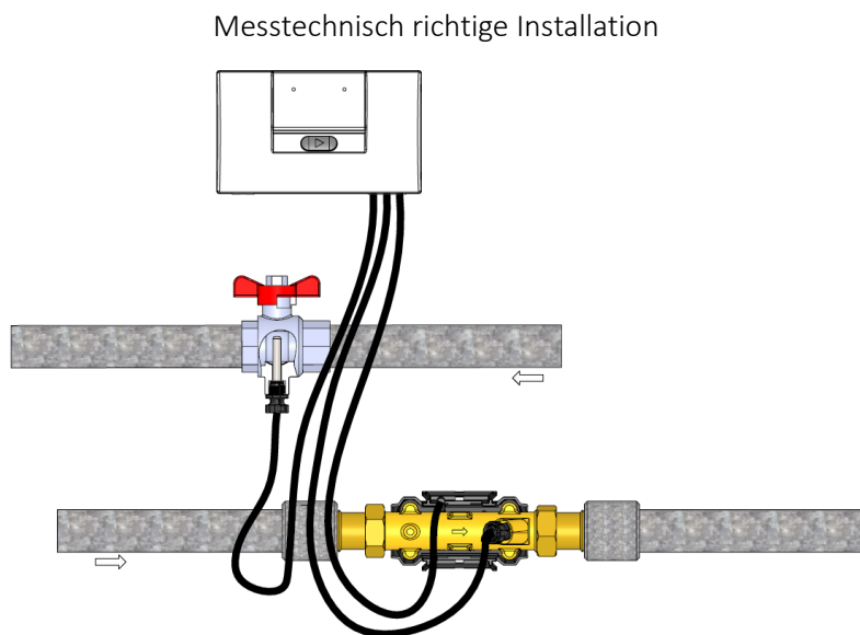
Abb. 23: Beispiel für eine messtechnisch richtige Installation.
