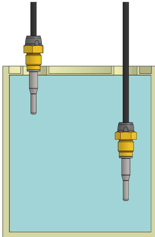
Abb. 18: Die qualifizierende Eintauchtiefe wird durch den Vergleich der Messungen an zwei Temperaturfühlern ermittelt, die vollständig und teilweise in das Wasser eingetaucht sind.
