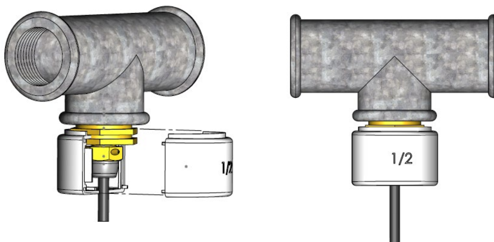
Abb. 30: Beispiele für das Plombieren von Temperaturfühlern, entweder mit Plombendraht oder mit Plombierschellen.
