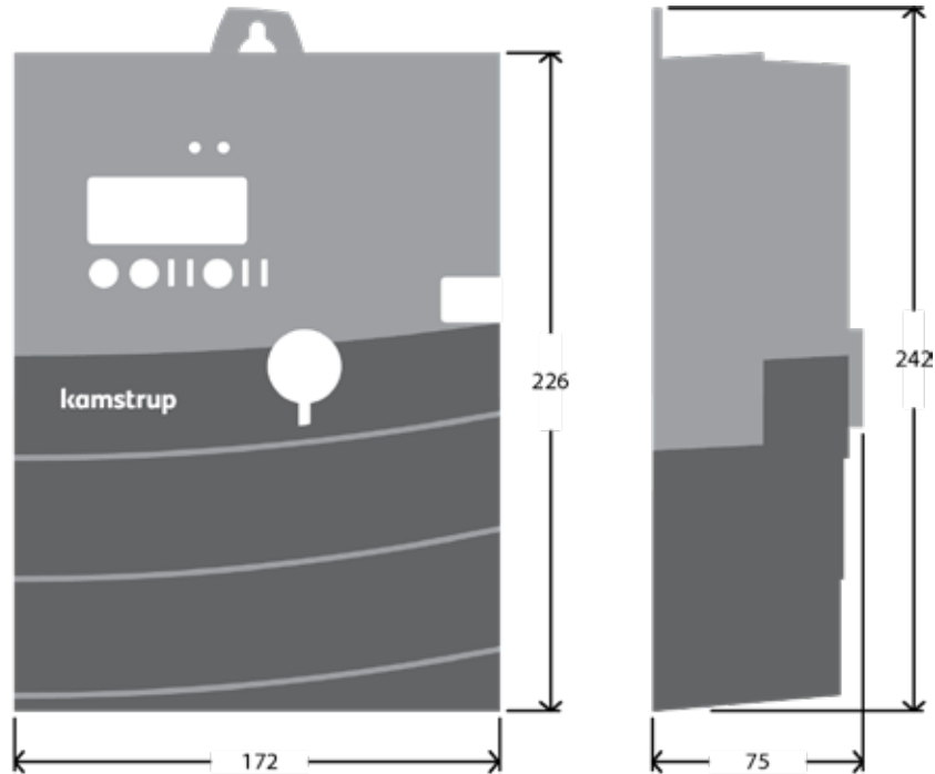
CT-Zähler 60 mm Klemmabdeckung
