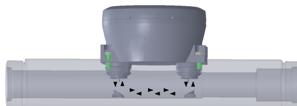
Ultraljudsprincipen
