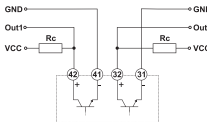
Fig. 21 Sorties statiques, référence GND
