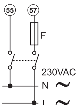
Fig. 18 Option D. F = 250 V, 50 mA
