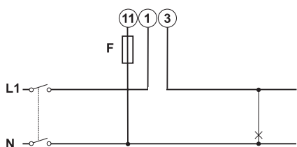
Fig. 15 AV2, AV9 (sauf IS, R2)
