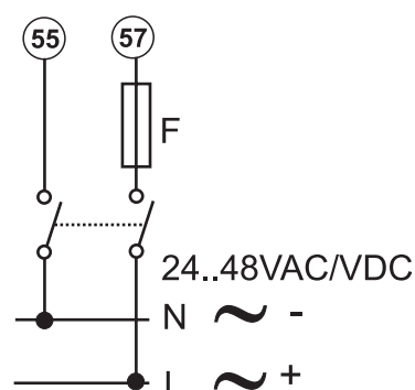
Fig. 20 Option L. F = 250 V, 200 mA
