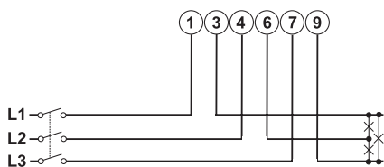
Fig. 5 AV2, AV9 (sauf IS, R2)
