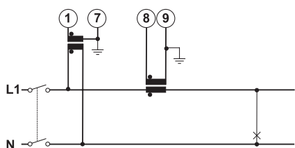
Fig. 15 AV2, AV9 (sauf IS, R2)
