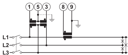
Fig. 11 AV6 charge équilibrée
