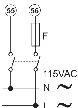
Fig. 19 Option D. F = 250 V, 100 mA
