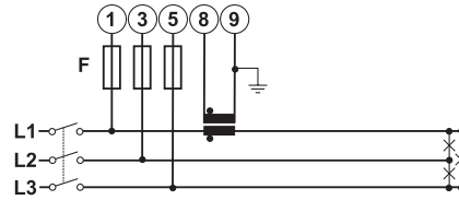
Fig. 10 AV5, AV6 charge équilibrée
