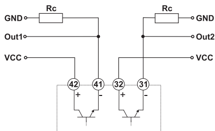
Fig. 22 Sorties statiques, référence VCC
