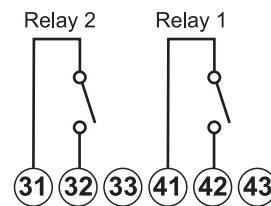
Fig. 23 Sorties à relais
