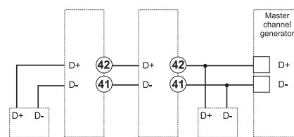
Fig. 26 Port Dupline
