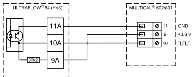
Схема 2 – Соединение трехжильным кабелем, MULTICAL® 602/801 через выходной модуль (Y=3).
