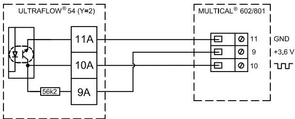
Схема 1 – Соединение трехжильным кабелем, MULTICAL® 602/801 через выходной модуль (Y=2).
