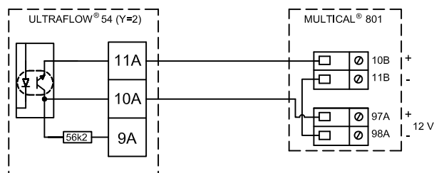
Схема 3 – Соединение двухжильным кабелем, MULTICAL® 801 через выходной модуль (Y=2).
