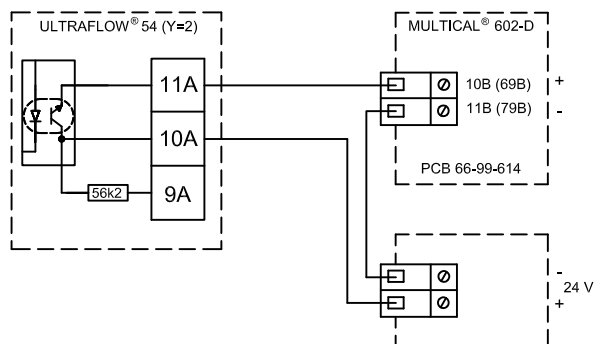
Схема 4 – Соединение двухжильным кабелем, MULTICAL® 602-D через выходной модуль (Y=2) и внешнее питание 24 В DC.
