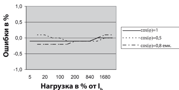
Кривая нагрузки
